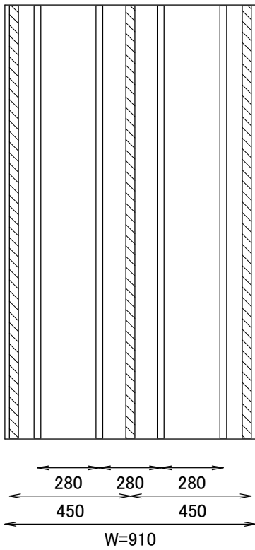
壁面施工例 (単位:mm)
