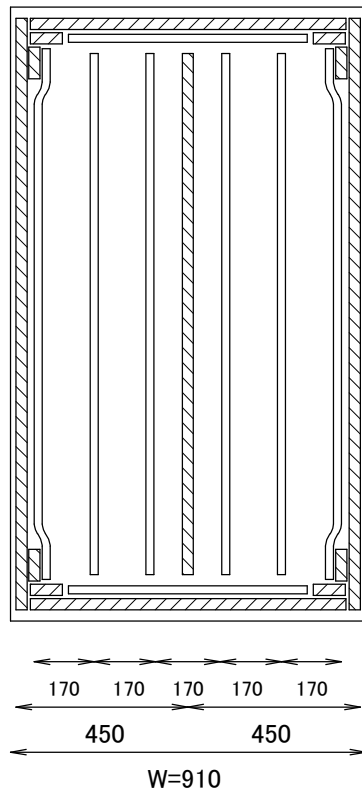
反りが大きい場合の施工例 (単位:mm)
